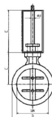
Typ GD-6 s montážní přírubou DIN/ISO
