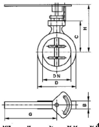
Typ GD-6 Plynulé nastavení typu RDST-32
