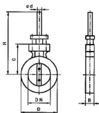
Typ GD-6 s volným hřídelem
